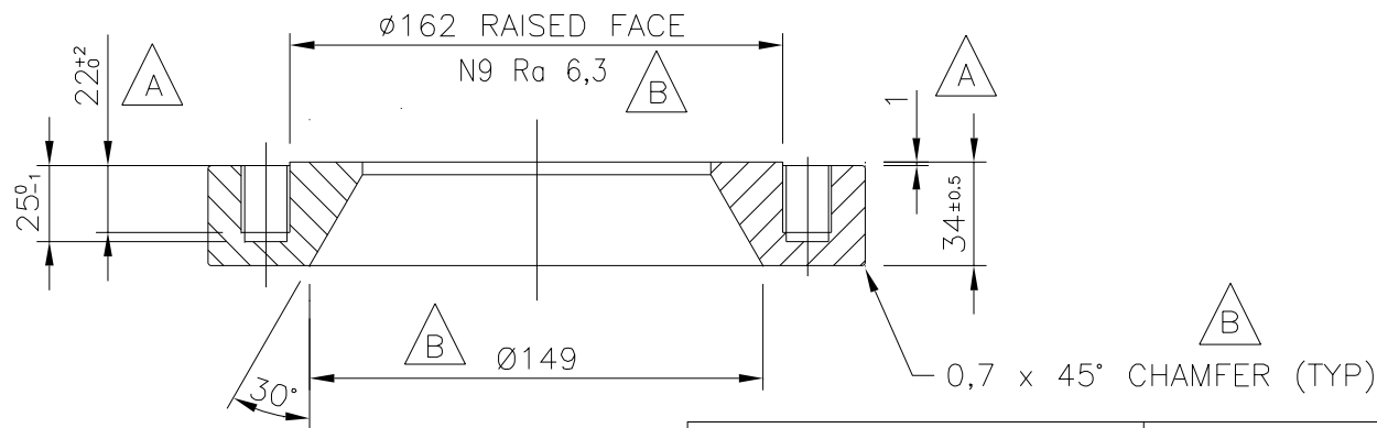
SECTION A-A SCALE 1:2
