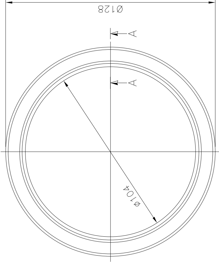
PLAN SCALE 1:1
